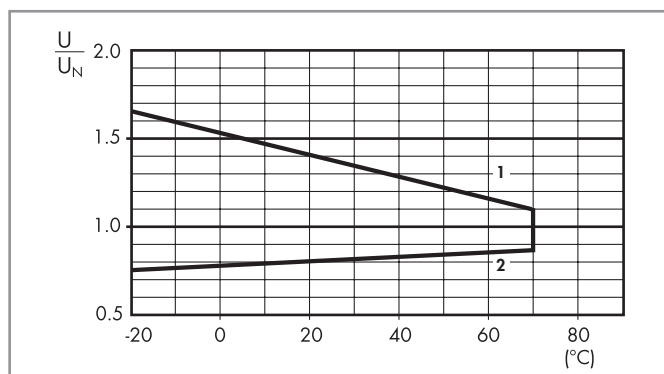
R 48 – 交流线圈工作范围对比环境温度
