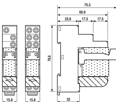
48.31 48.52 / 48.61 / 48.62 螺丝端子
